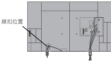
方式 2 (腳座安裝於內側時)
