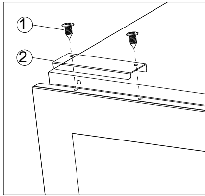
i42SBTIH/i42SSTIH/i46DBTIH/i46SBTIH 把手安裝示意圖
