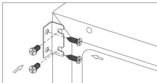
固定支架安裝示意圖
