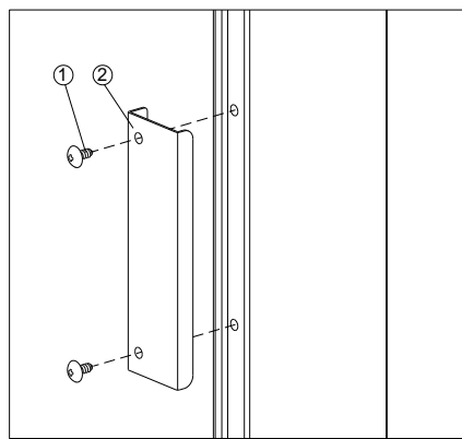
i170DBTIH/i180DBTIH/i180DSTIH 把手安裝示意圖
